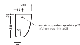
sezione longitudinale / section
