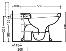
sezione longitudinale / section
