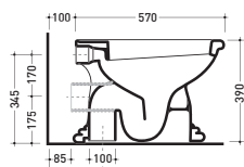
sezione longitudinale / section
