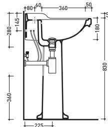
sezione longitudinale / section
