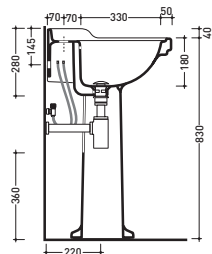
sezione longitudinale / section
